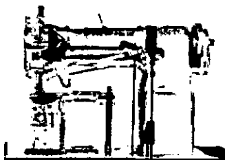
Marca: DÜRKOPP ADLER AG Especialidad: Horta manga País de origen: Alemana Período de fabricación: Años 80 Modelo: Typ 0541 015103 Descripción: Para usar las mangas en los delanteros y traseros de las prendas de vestir (abacos, chaquetas, entre otras)
